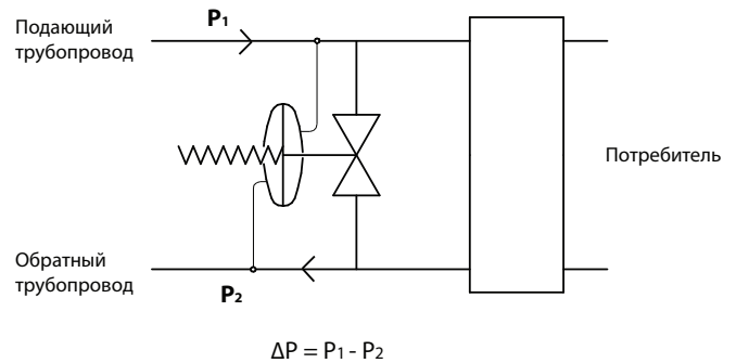
Рис. 3. Установка на байпасе к потребителю
