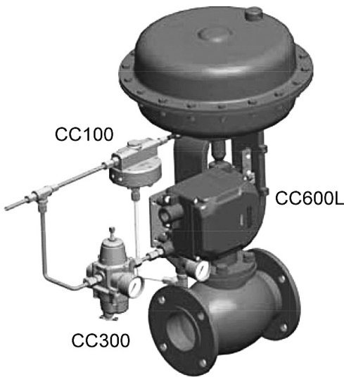
Привод одностороннего действия
