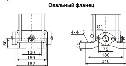
Варианты подключения ВМНч II
