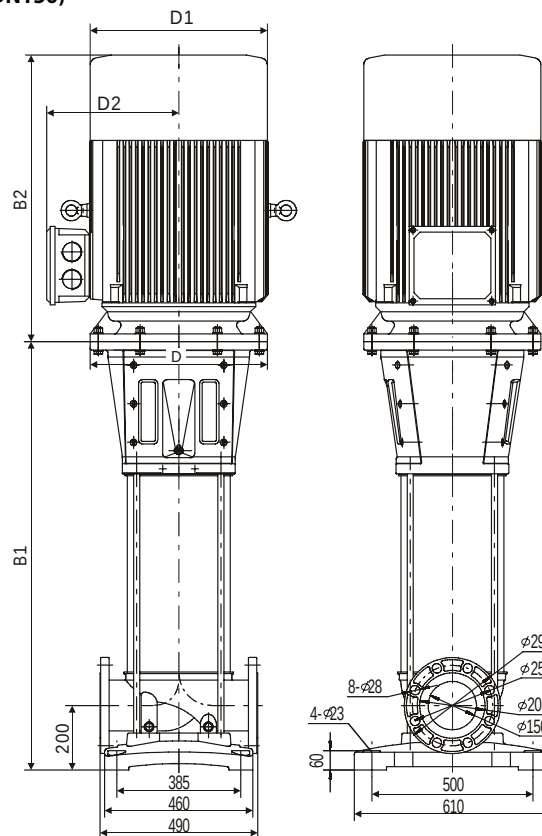
Круглый фланец PN25-40(DN150)
