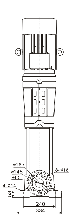
Вариант подключения ВМНч II
