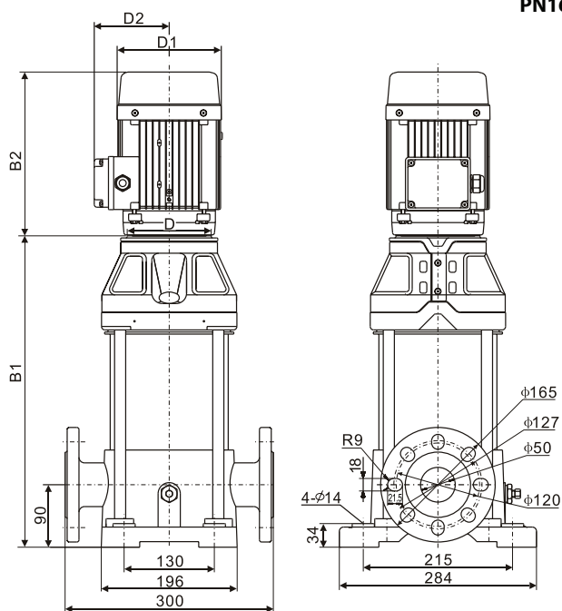
Вариант подключения ВМНч II
