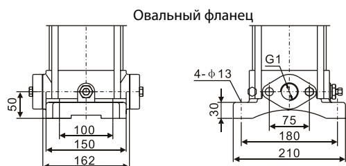
Варианты подключения ВМНч II
