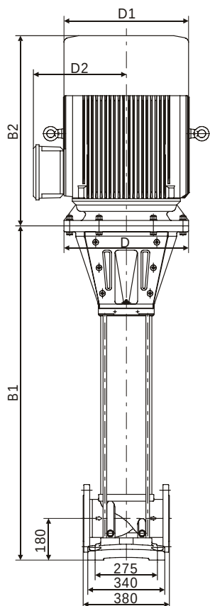
Варианты подключения ВМНч II
