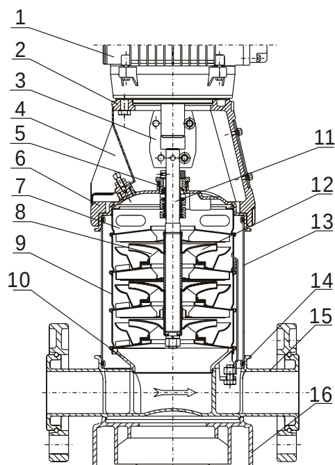
ВМН 10,15,20 II
