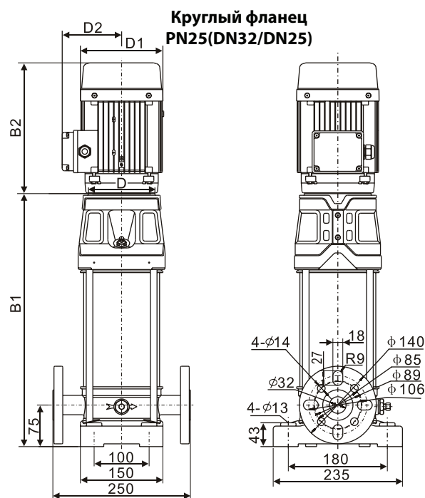
Вариант подключения ВМН II
