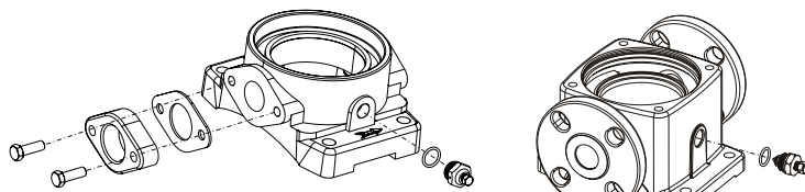
Овальный фланец
