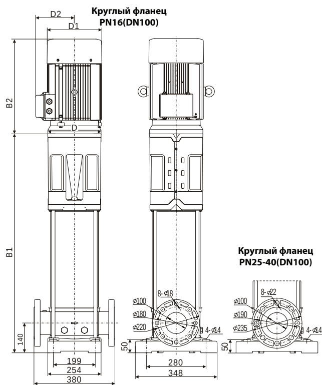
Варианты подключения ВМН II
