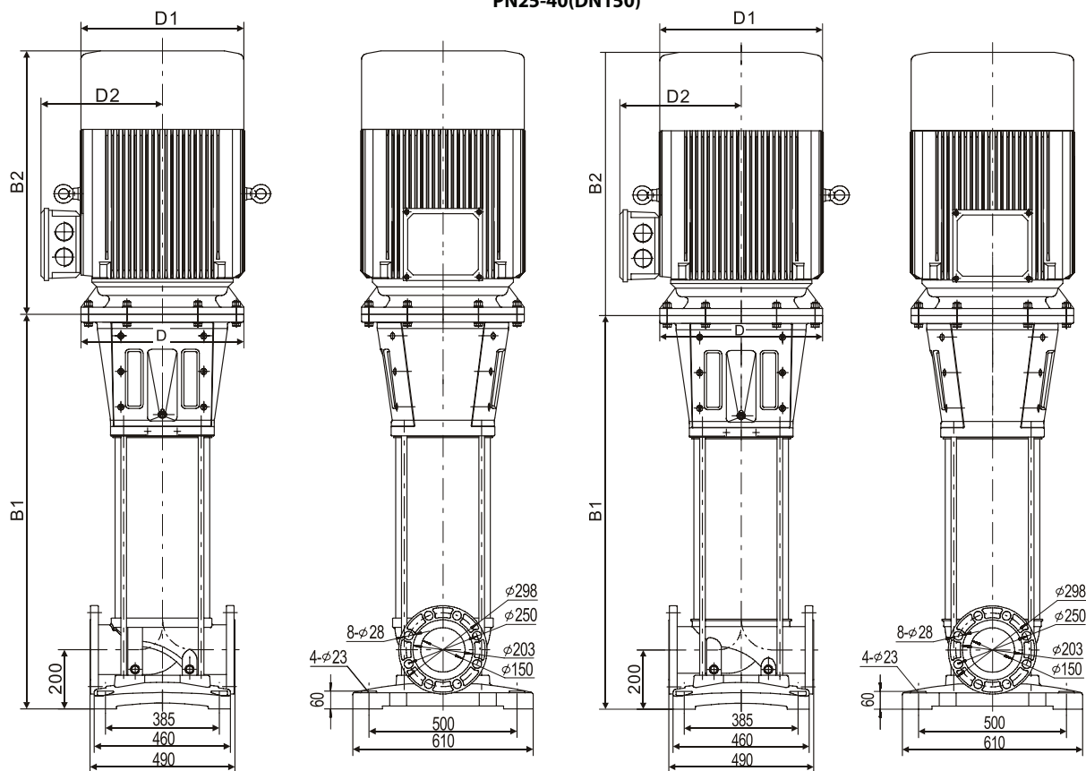
Круглый фланец PN25-40(DN150)
