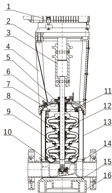
ВМН 32,45,64,90 II
