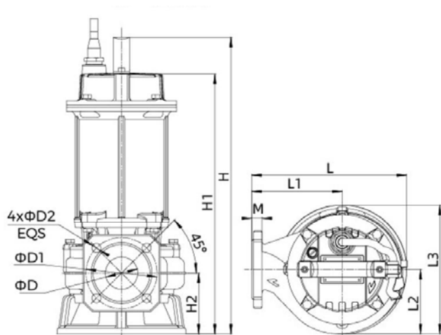
Однофазное исполнение
