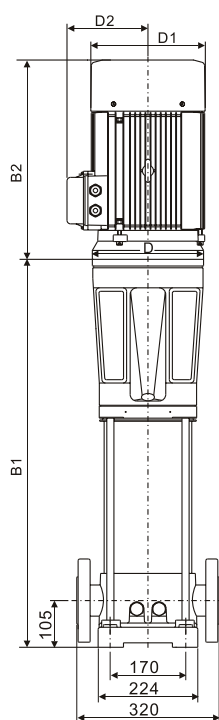
Вариант подключения ВМНч II
