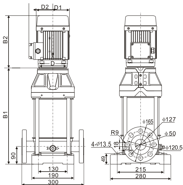
Круглый фланец PN16-25-40(DN50)
