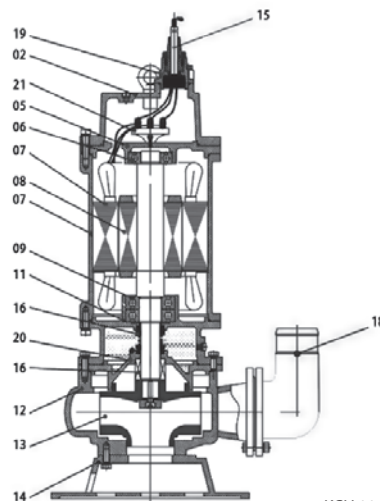
КСН 11-45 кВт
