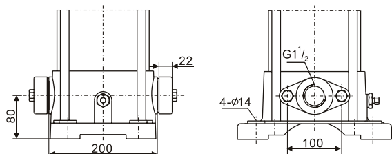
Овальный фланец
