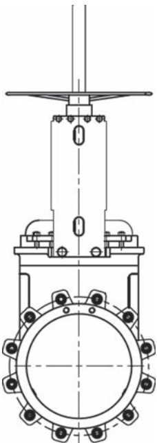
Штурвал с выезным штоком
