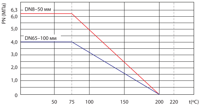
Диаграмма «Температура-Давление»
