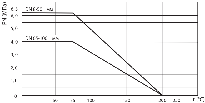
Диаграмма «Температура-Давление»
