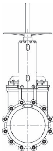
Штурвал с выезным штоком
