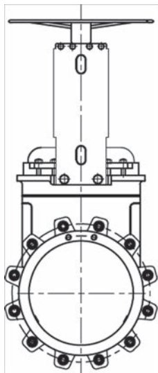
Штурвал с невыезным штоком
