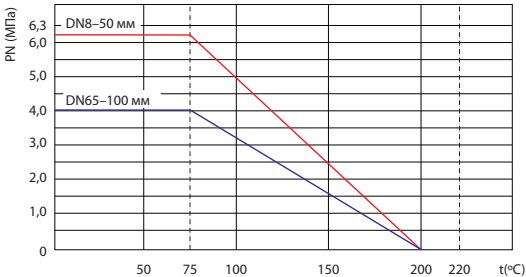
Диаграмма «Температура-Давление»
