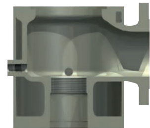
Паровая рубашка
