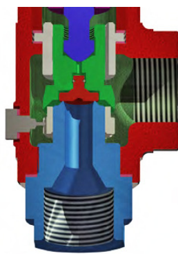
Внутренняя резьба
