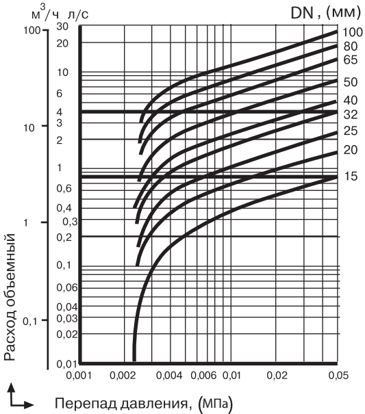
Диаграмма падения давления на клапане
