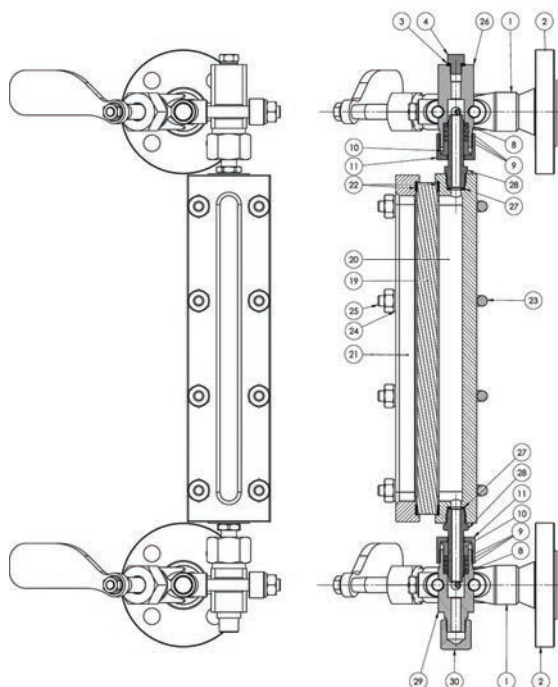
Спецификация корпуса указателя СТИМЛЕВЕЛ «РС»
