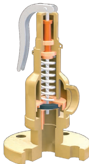
Предохранительный клапан
