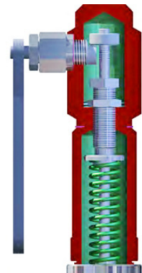
Подрывной рычаг
