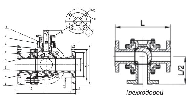
Трехходовой
