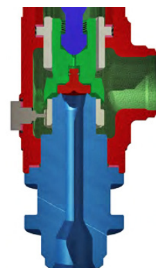
Приварка встык
