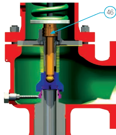
Сильфонно-плунжерный клапан
