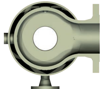
Паровая рубашка
