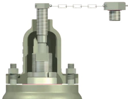
Испытательная заглушка
