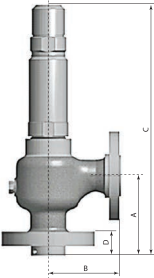
Фланцевое присоединение
