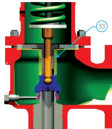
Сильфонный клапан
