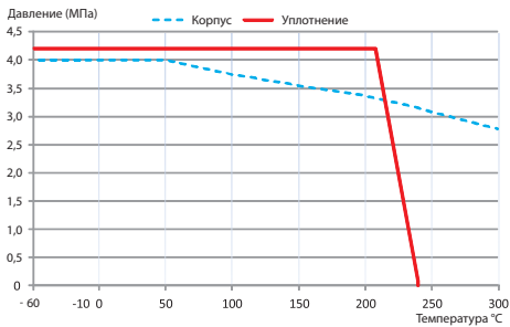
Диаграмма «Температура-Давление»
