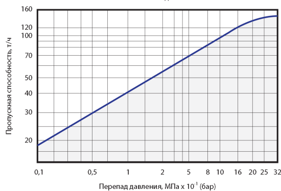
Расход
