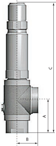
Внутренняя резьба
