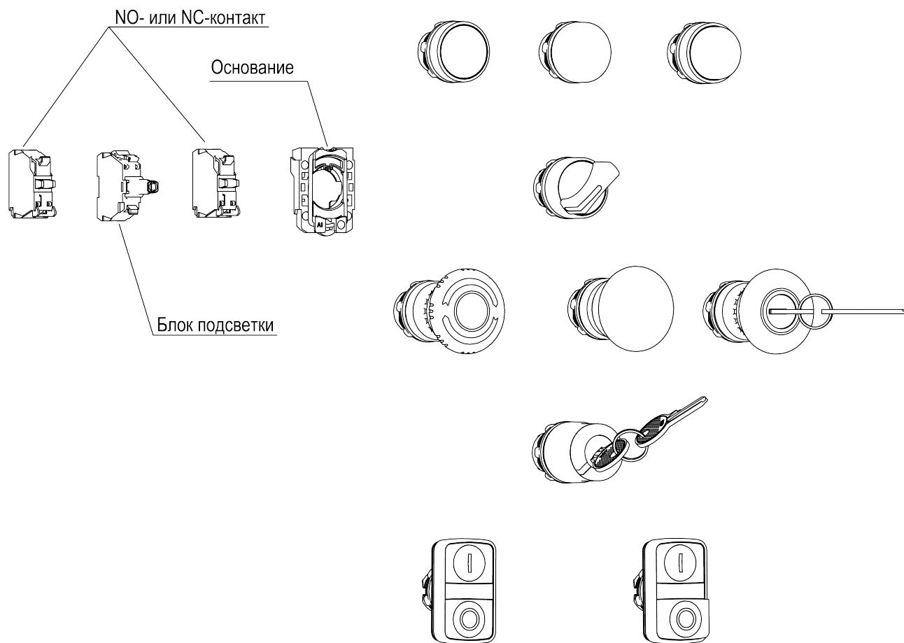
Рисунок 4.1 – Конструкция
