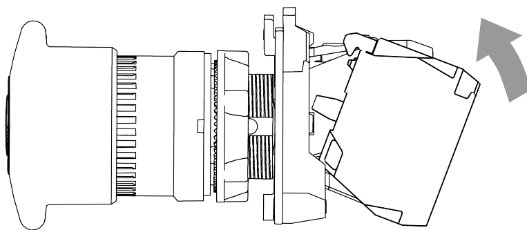
Рисунок 6.5 – Монтаж блок-контакта
