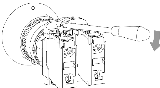
Рисунок 6.2 – Отсоединение головки
