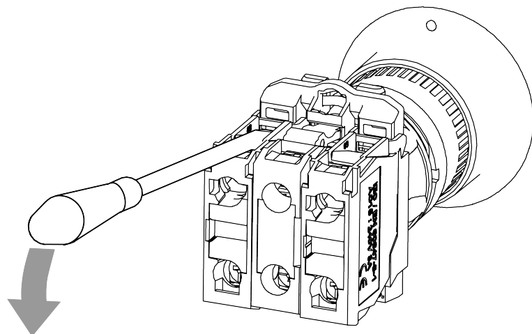
Рисунок 6.6 – Демонтаж блок-контакта
