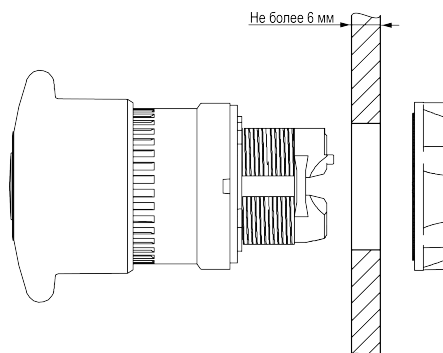
Рисунок 6.3 – Установка в щит
