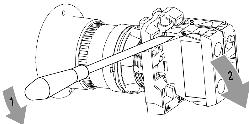
Рисунок 6.7 – Демонтаж блока подсветки
