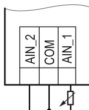
Рисунок 6.7 – Подключение резистивных датчиков
