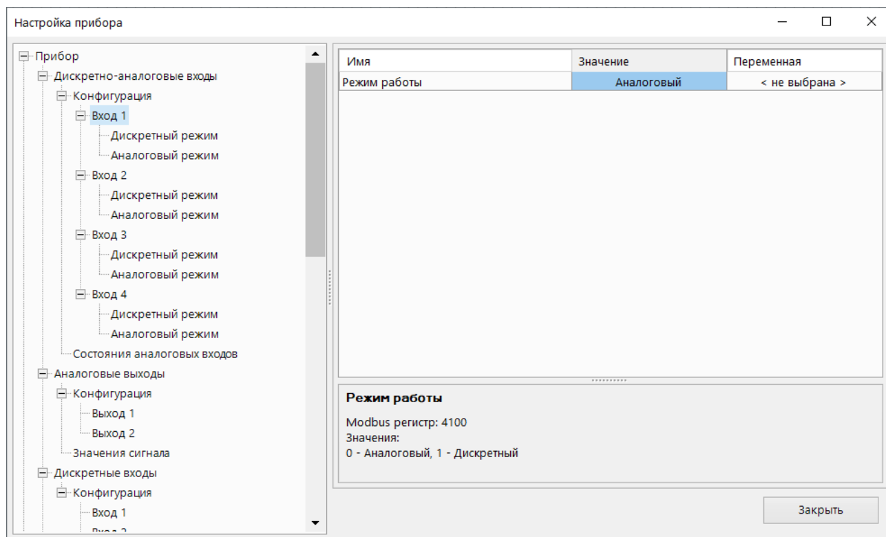
Рисунок 4.1 – Настройка режима работы входа типа «TRM»
