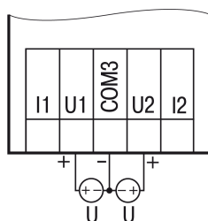
Рисунок 6.18 – Подключение датчиков с выходом в виде напряжения
