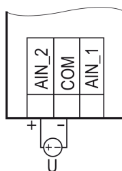
Рисунок 6.5 – Схема подключения датчиков с выходными сигналами постоянного напряжения и от 0 до 1 В и от 0 до 10 В
