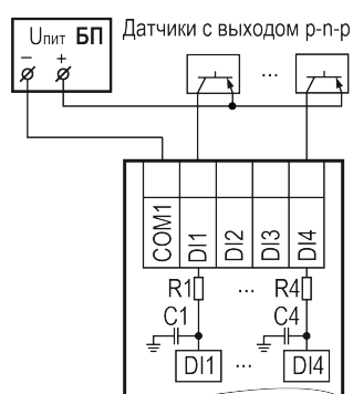
Рисунок 6.13 – Подключение к входам типа «Д» датчиков с выходом р-п-р
