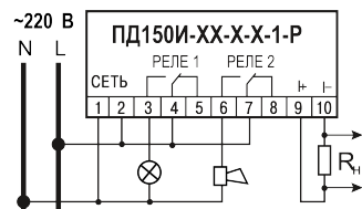
Рисунок 2 – Пример схемы подключения
