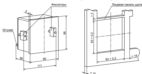
Рисунок 1 – Габаритные и установочные размеры преобразователя щитового исполнения
