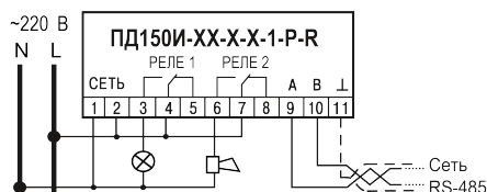
Рисунок 2 – Пример схемы подключения
